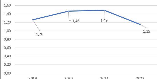
Indikátor: Teplo (GJ)/pracovník
